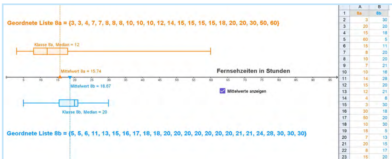
Abb. 17. Boxplot und Mittelwert © GeoGebra, ELSCHENBROICH & DUTKOWSKI
