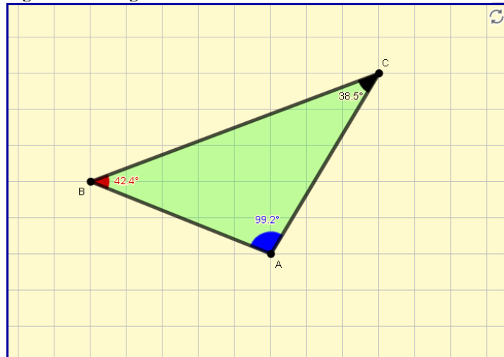
Figura 1 – Triângulo ABC
