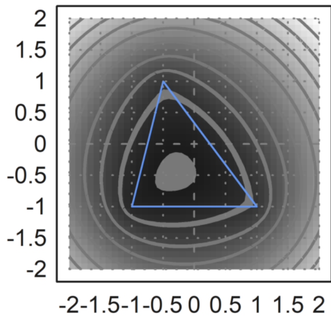
The Fermat point
