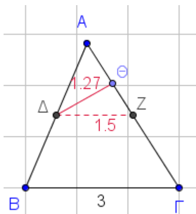
Μοντέλο του προβλήματος στο Geogebra
