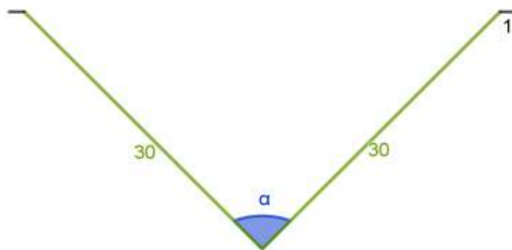
Figura 1 – Planificação da calha seção triangular
